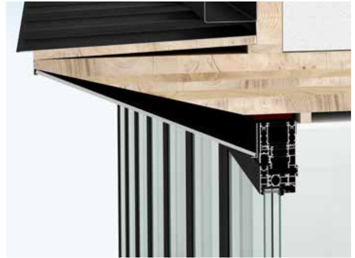
Anschlussmöglichkeit Glas-Faltwand
